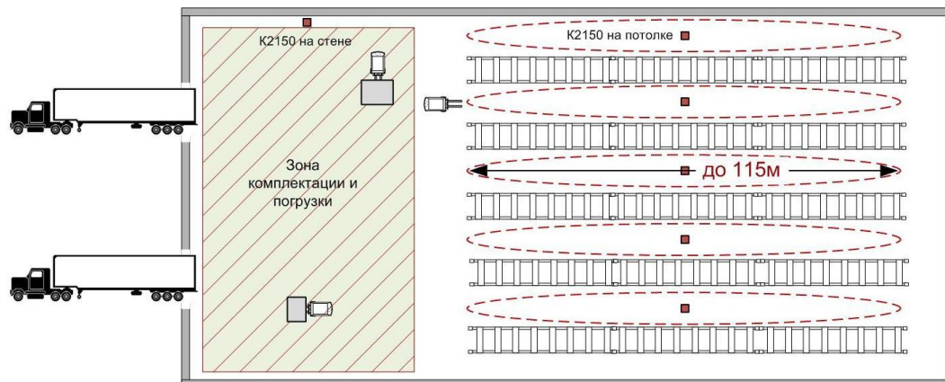
Схема организации системы автоматического управления освещением склада
