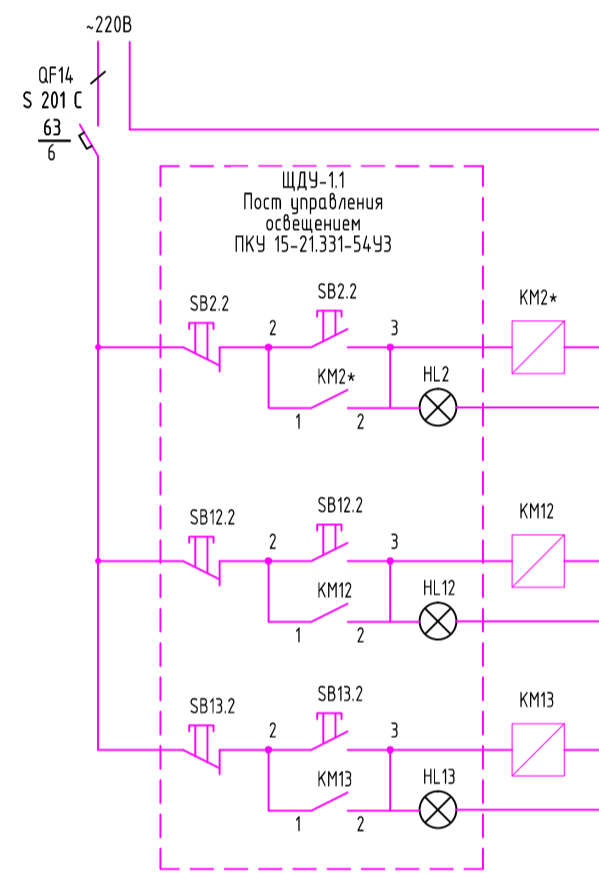
Фрагмент схемы электрической принципиальной ручного управления освещением.
