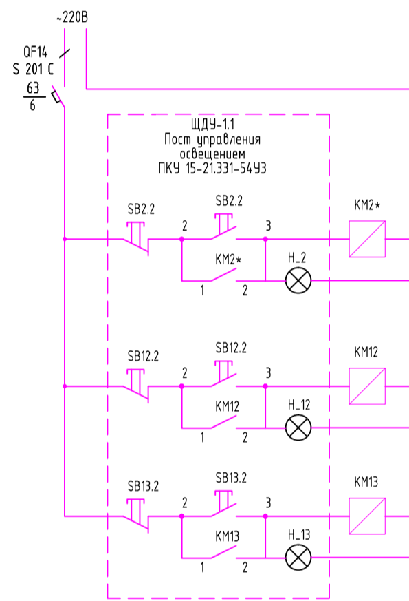
Фрагмент схемы электрической принципиальной ручного управления освещением.
